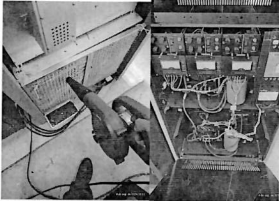
Mantenimiento al transmisor de FM y regulador de voltaje en caseta de transmisión
